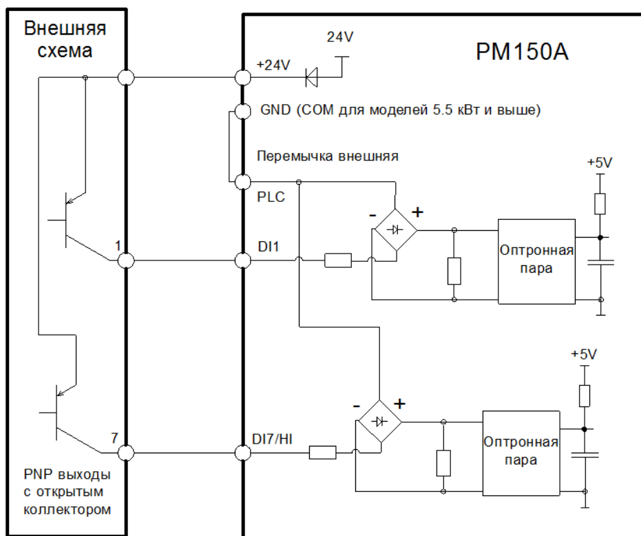
(а) с использованием внутреннего источника питания
