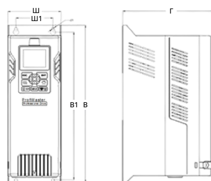
Габаритные размеры преобразователей мощностью 5,5 ~ 7,5 кВт
