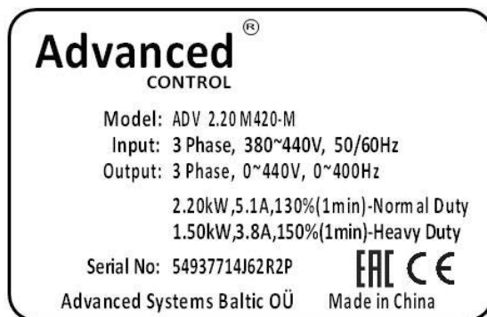
Рис. 2-2. Заводская табличка
