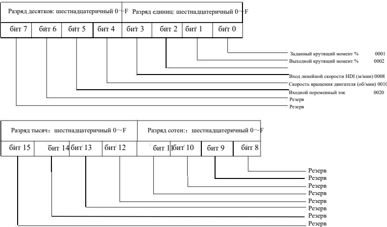
Рис. 5-20. Индикация на LED-дисплее при работе
