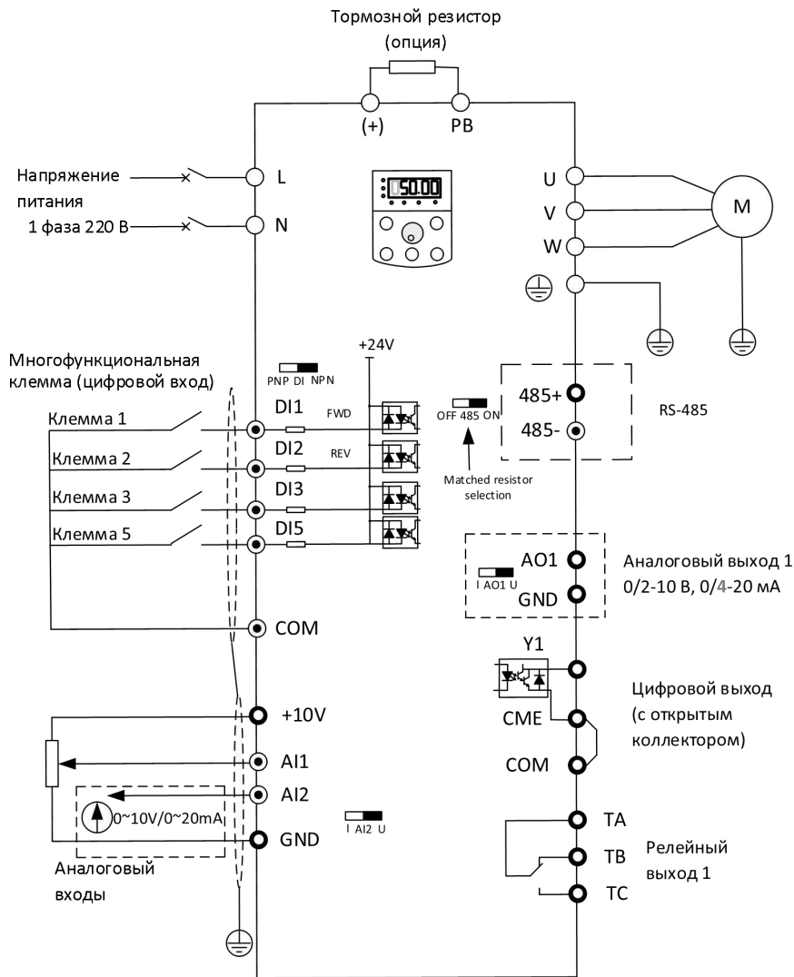
Рис. 3-3. Преобразователи частоты до 1,5 кВт (220 В) (включительно) ADV 0.40 M220-M ~ ADV 1.50 M220-M (0.4~1.5 кВт)
