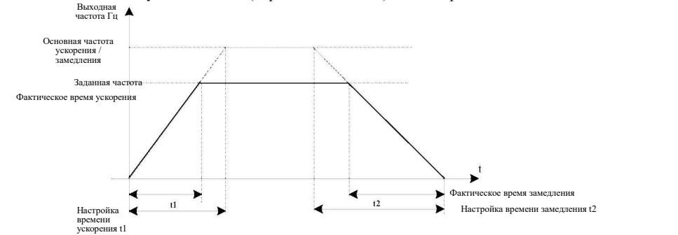
Рис. 5-2. Иллюстрация времени ускорения / замедления
