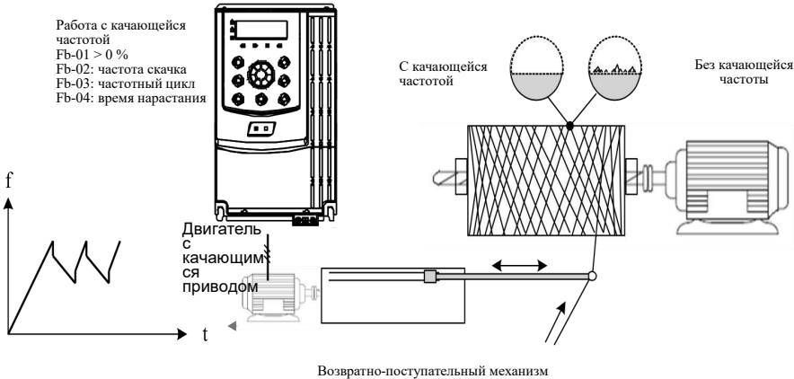
Рис. 4-20 Иллюстрация применения режима качающейся частоты.
