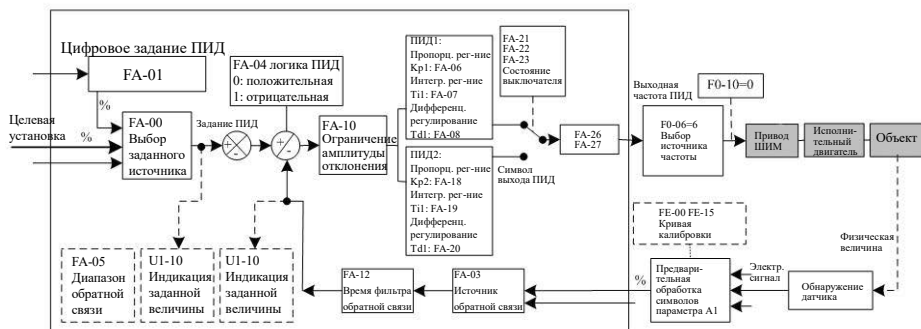
Рис. 4-19. ПИД-регулирование частоты с обратной связью.
