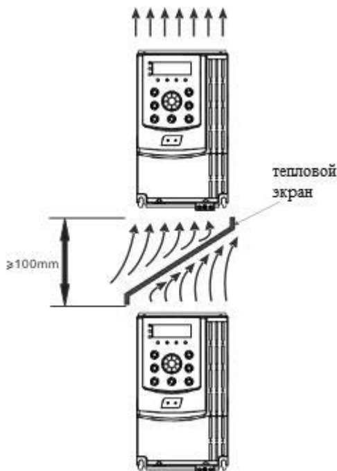
Рис. 3-1. Иллюстрация монтажа M220/M420
