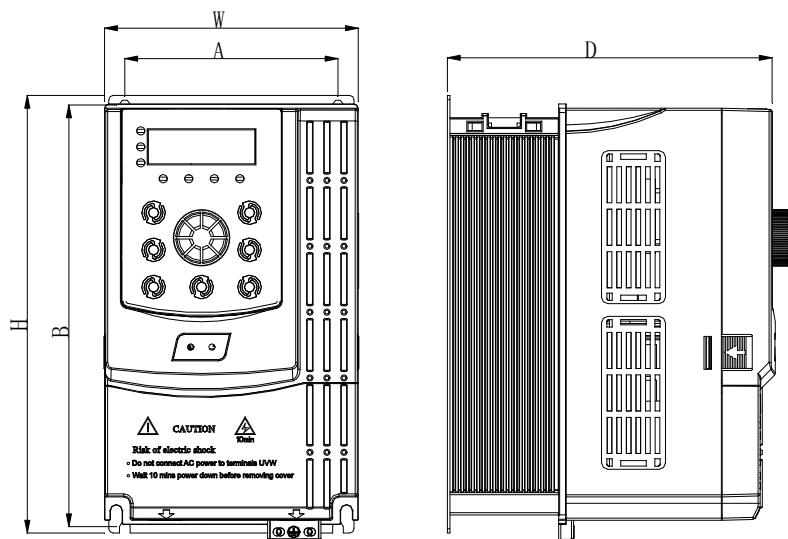
Рис. 2-4 Габаритные и монтажные размеры корпуса преобразователя из пластмассы (до 18.5 кВт)
