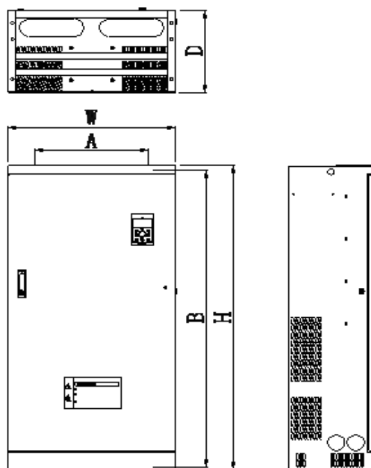
Рис.2-7 Габаритные и монтажные размеры корпуса преобразователя свыше 185 кВт
