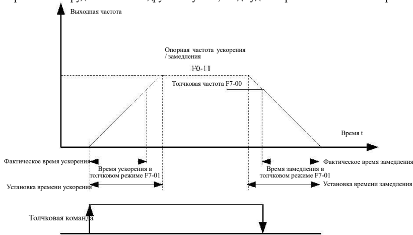
Рис. 4-14. Иллюстрация толковой режима работы
