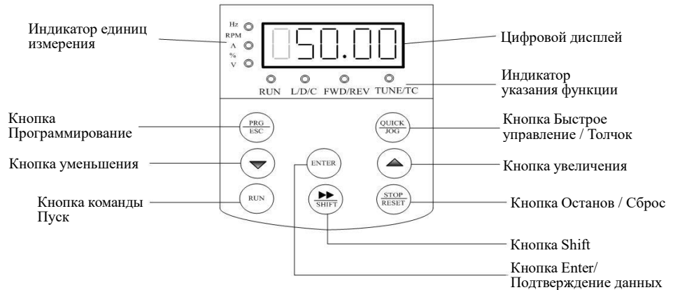
Рис. 4-2. Пульта управления 2
