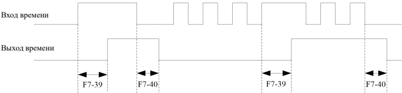
Рисунок 5-19. Диаграмма работы входа и выхода таймера
