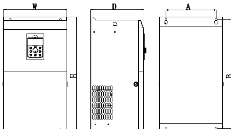
Рис.2-6 Габаритные и монтажные размеры корпуса преобразователя 55-160 кВт
