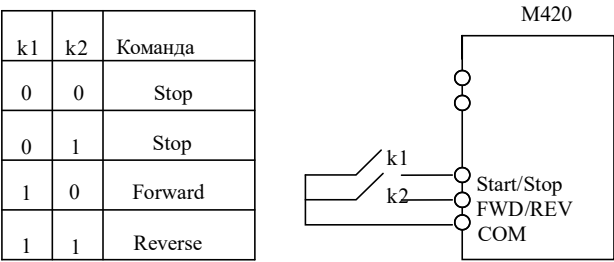
Рис. 5-8. Двухпроводный режим управления 2
