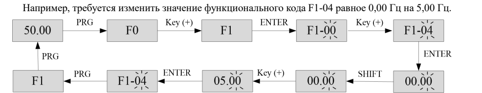
Рис. 4-3. Блок-схема установки параметра
