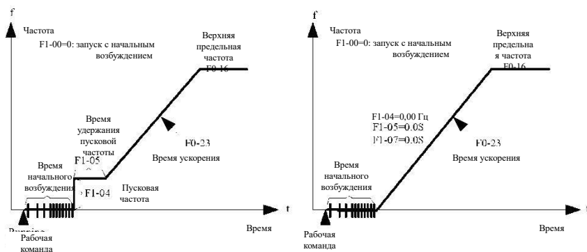
Рис. 4-12. Иллюстрация запуска с начальным возбуждением
