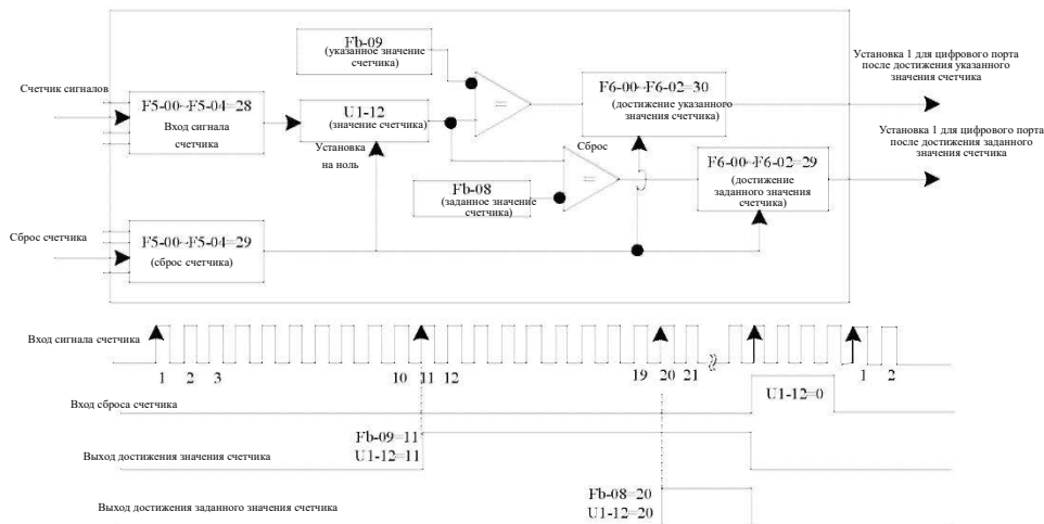
Рис. 4-25. Установка функционального кода в режиме счетчика
