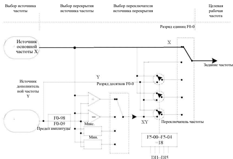
Рис. 5-1. Иллюстрация наложения источников частоты.
