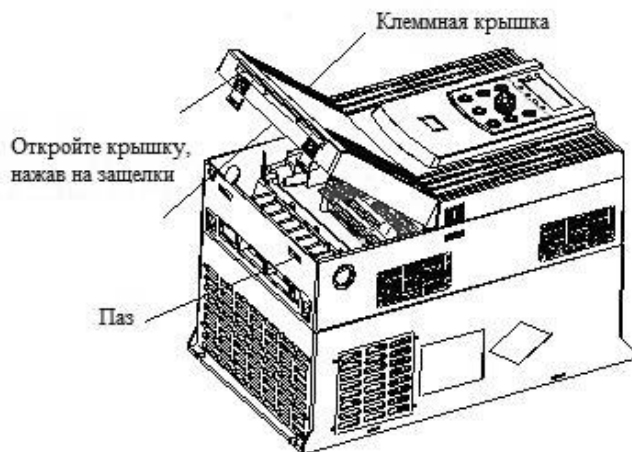
Рис. 3-2. Снятие верхней крышки пластмассового кожуха
