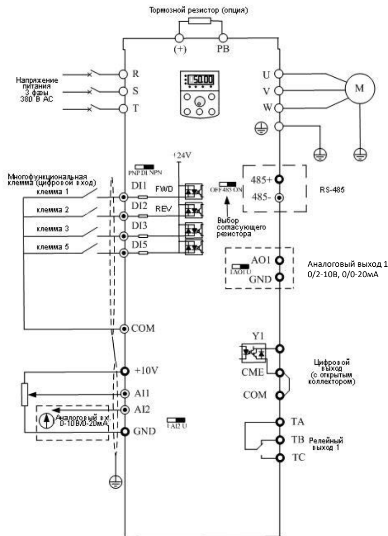
Рис. 3-5. Преобразователи до 2,2 кВт (380 В) (включительно)
