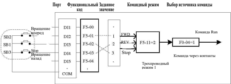
Рис. 4-9. Иллюстрация режима управления запуск-останов через клеммы.
