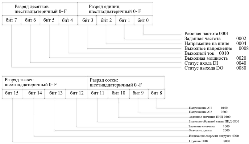
Рис. 5-17. Индикация на дисплее при работе
