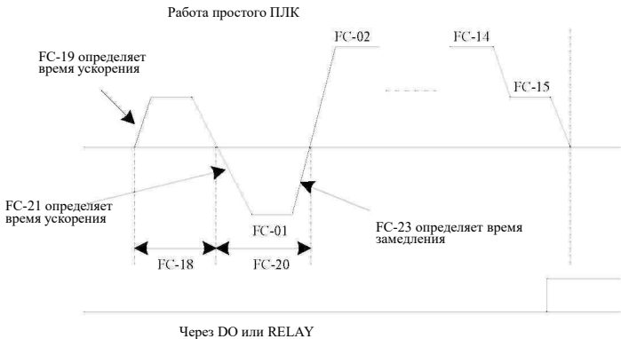
Рис. 5-28. Иллюстрация простого ПЛК
