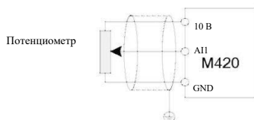
Рис. 3-9. Принципиальная схема для подключения входного клеммам аналогового сигнала.
