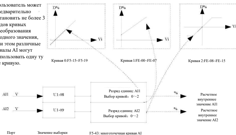
Рис. 4-28. Фактическое задание сигнала AI
