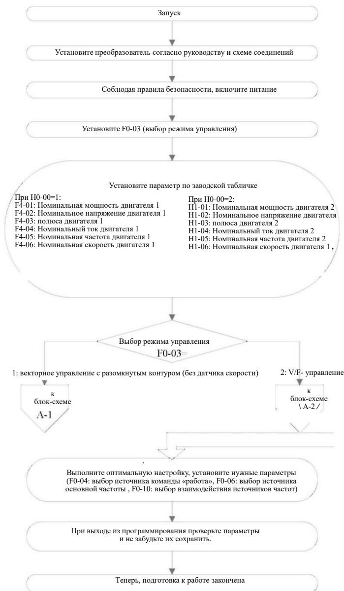
Рис. 4-5. Основные шаги перед началом работы
