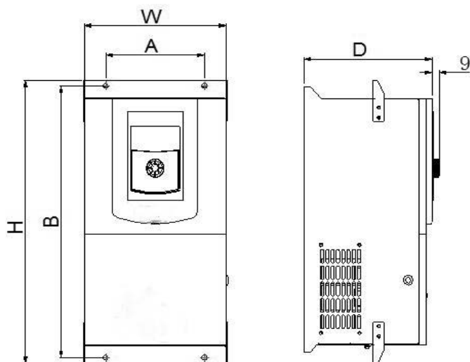
Рис.2-5 Габаритные и монтажные размеры корпуса преобразователя из металла (22-45 кВт)
