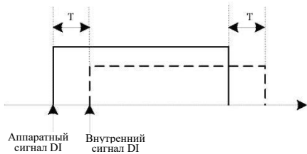
Рис. 4-27. Настройка задержки срабатывания входа DI.
