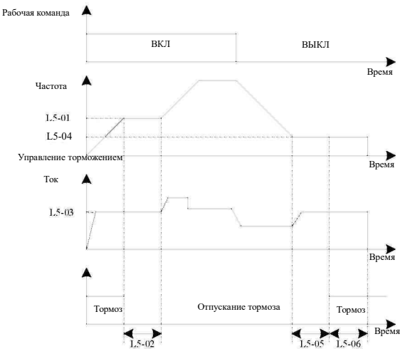
Рис. 5-30. Иллюстрация ленточного процесса торможения
