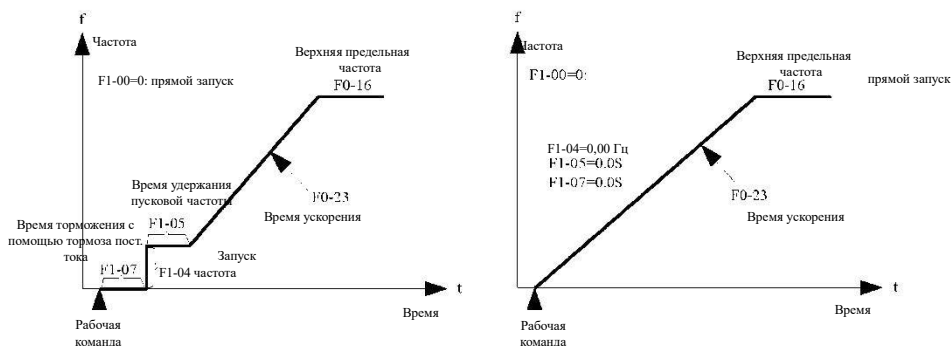
Рис. 4-11. Иллюстрация прямого запуска
