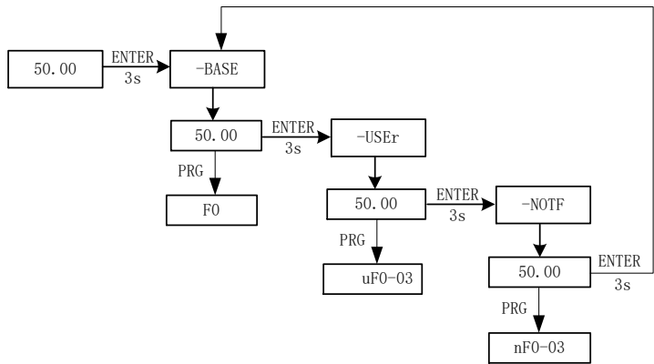
Рис. 4-4. Рабочая схема переключения режима меню
