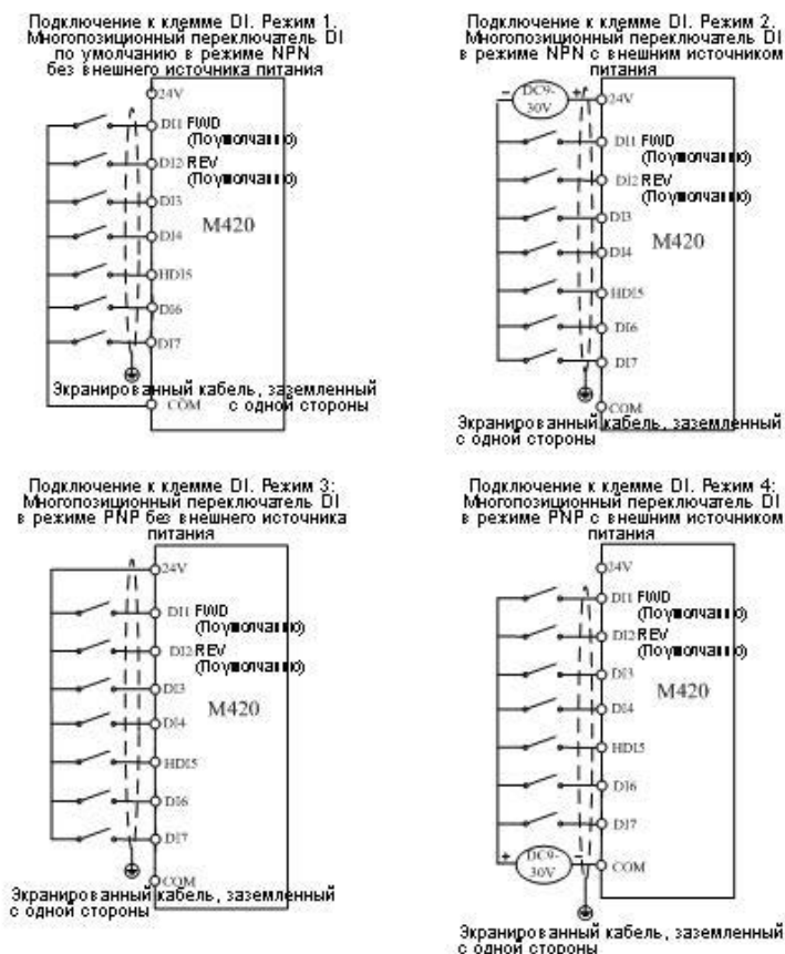
Рис. 3-10. Четыре различных схемы подключения.
