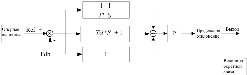
Рис. 5-22. Блок- схема ПИД - регулирования
