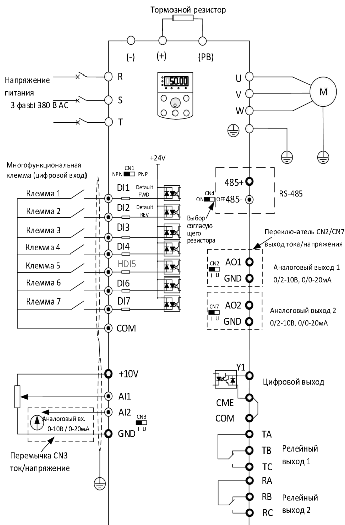
Рис. 3-6. Преобразователи от 4 до 37 кВт, 380 В
