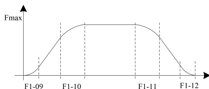
Рисунок 5-3. Иллюстрация S-кривой ускорения / замедления
