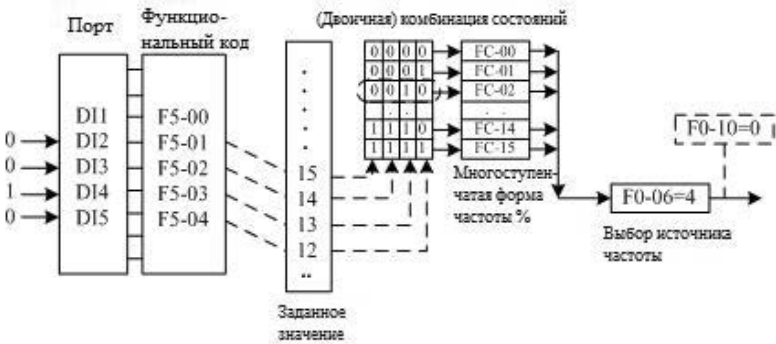
Рис. 4-21. Иллюстрация многоскоростного режима.
