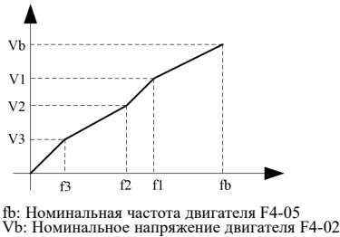
Рисунок 5-5. График V/F характеристики.
