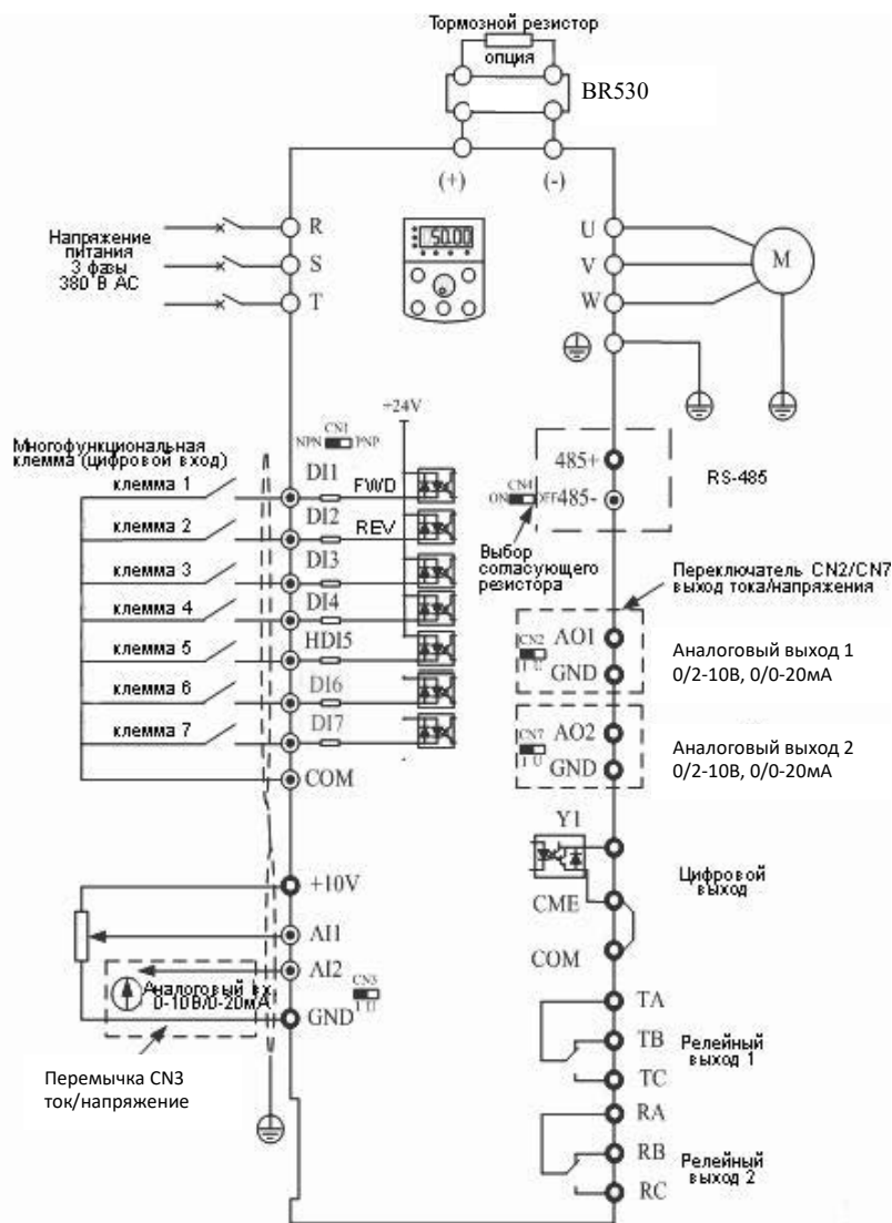
Рис. 3-7. Преобразователи частоты 2.2-5.5 кВт, 220 В / 45-75 кВт, 380В
