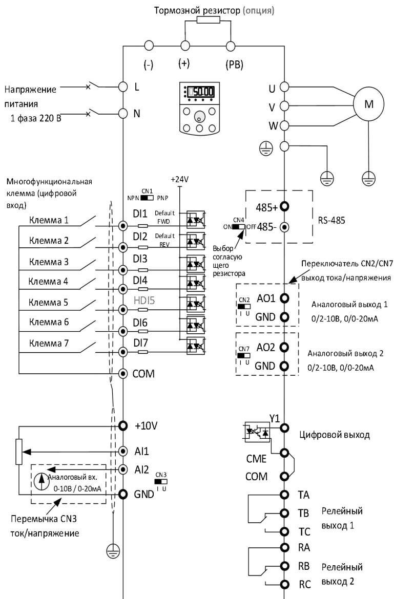
Рис. 3-4. Преобразователи частоты 2,2 - 5,5 кВт, 220 В
