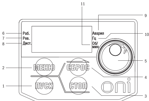
Рисунок 5.1.1. Кнопочная панель
