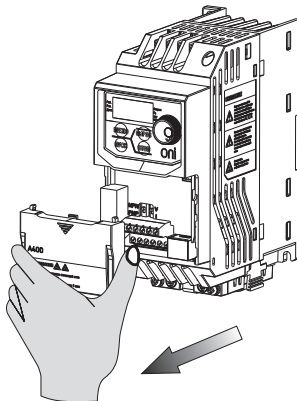
Шаг 2: снимите крышку клеммной колодки
